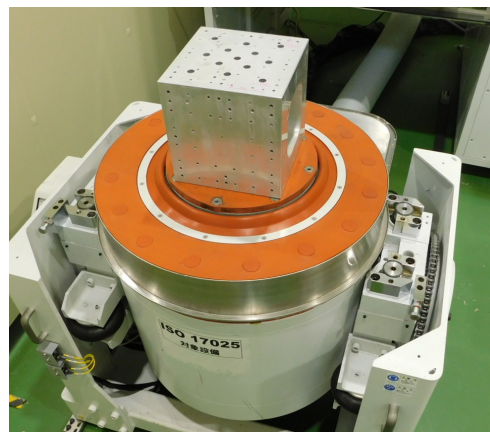
図 動電型振動試験機(加振力40 kN)
